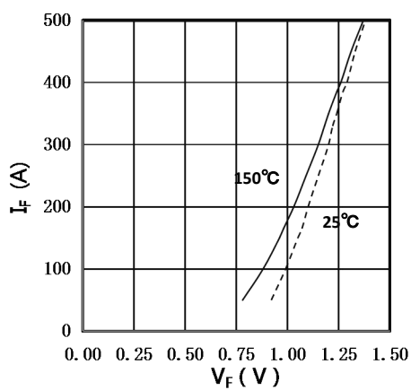
图3.压降特性曲线
