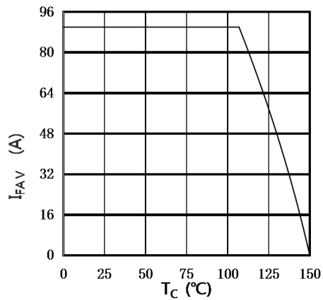
图1.壳温与电流特性曲线
