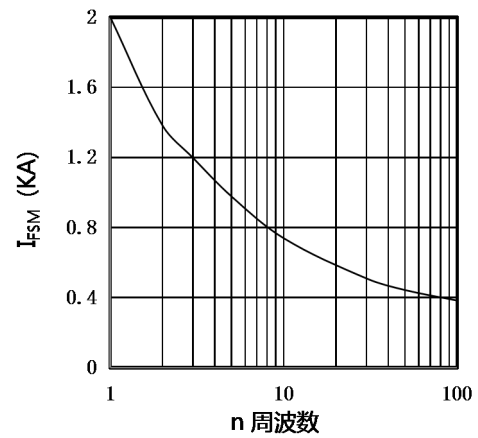
图4.浪涌电流特性曲线
