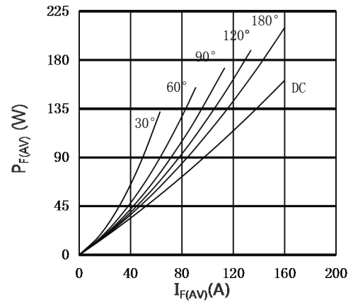
图2.平均功耗特性曲线
