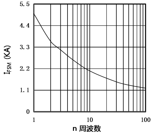
图4.浪涌电流特性曲线
